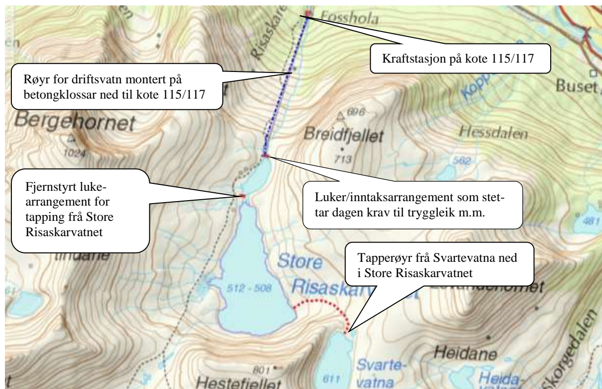
Figur 3. Kartutsnittet viser i grove trekk dei viktigaste naturinngrepa slik som inntak i Litlevatnet, røyrgate og kraftstasjon. Kraftstasjonen ligg aust for Risaskarrelva. Den stipla raude lina illustrerer tapperøyrte som er lagd mellom det fremste av Svartevatna og Store Risaskarvatnet for å sikre vassforsyninga til kraftverket og Vartdal vassverk i turre periodar. Denne er no planlagd at skal gjerast permanent, dvs at den skal gravast ned. Kartet er henta frå GisLink.
